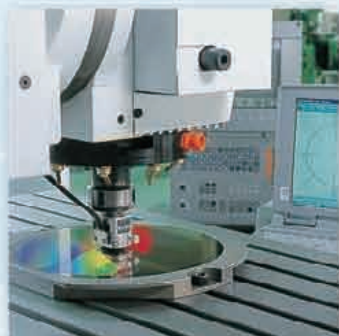
Prüfung des Bahnverhaltens einer CNC-gesteuerten Werkzeugmaschine
